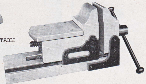
N° 98 ÉTAU PARALLÈLE A CHARIOT, VIS FER, POUR SCULPTEUR
